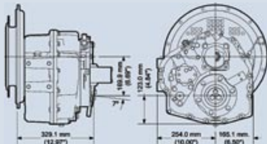
MG-5065 A (DOWN ANGLE)
